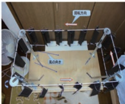
世界初、ループ式風力デモ機(半固定式)
