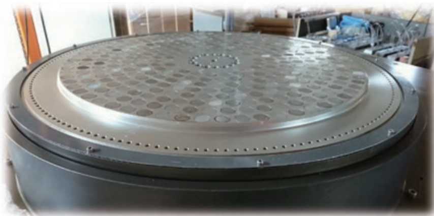
MAGHEAT1 号機の磁石盤
