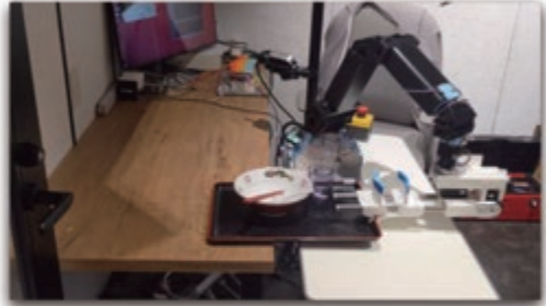
試作2号機：お盆の下膳
