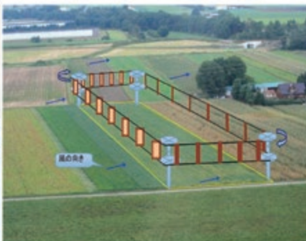
世界初、営農型風力発電
