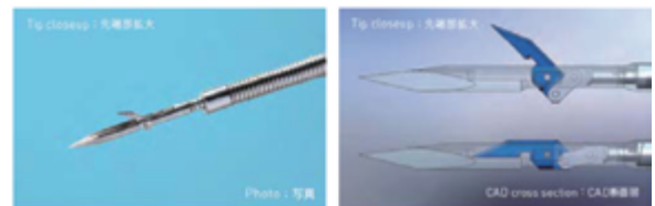
日本の精密加工技術を使った医療機器試作例(φ1.1mm)
